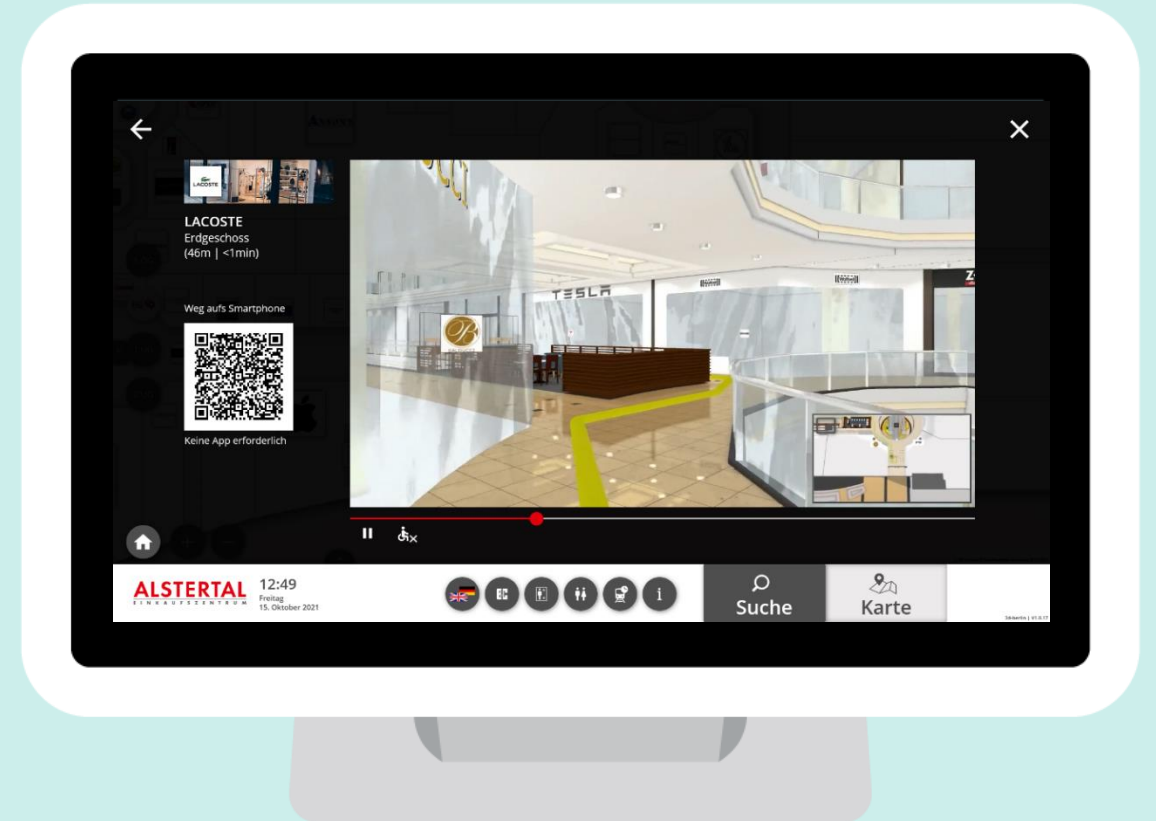
3D-Wegführung
