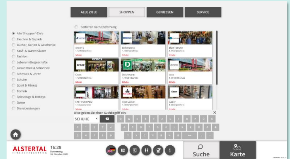
Kategorie & Stichwortsuche
