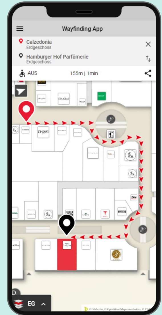
Weganzeige
