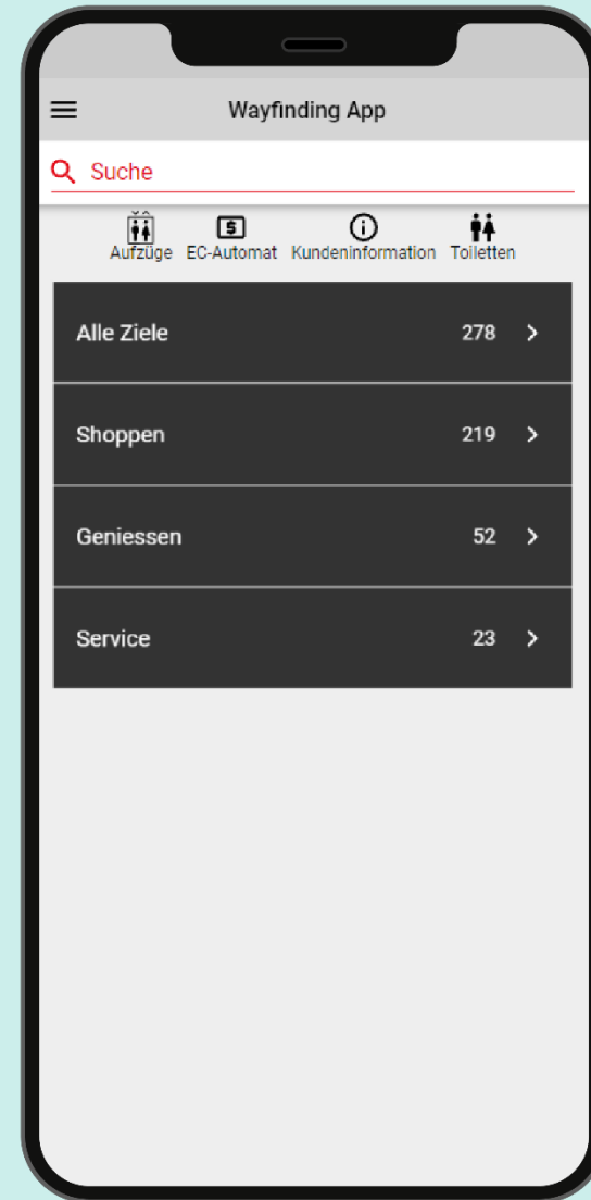
Suche
