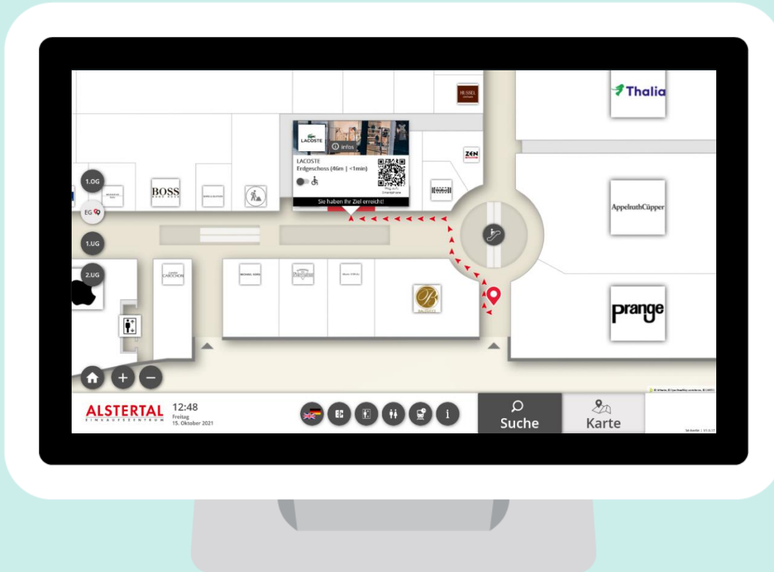
2D-Wegführung
