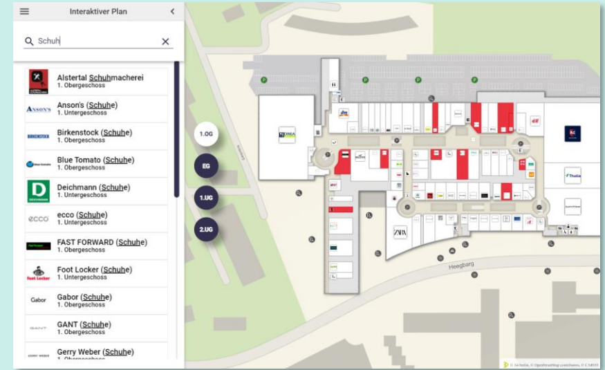
Stichwortsuche
