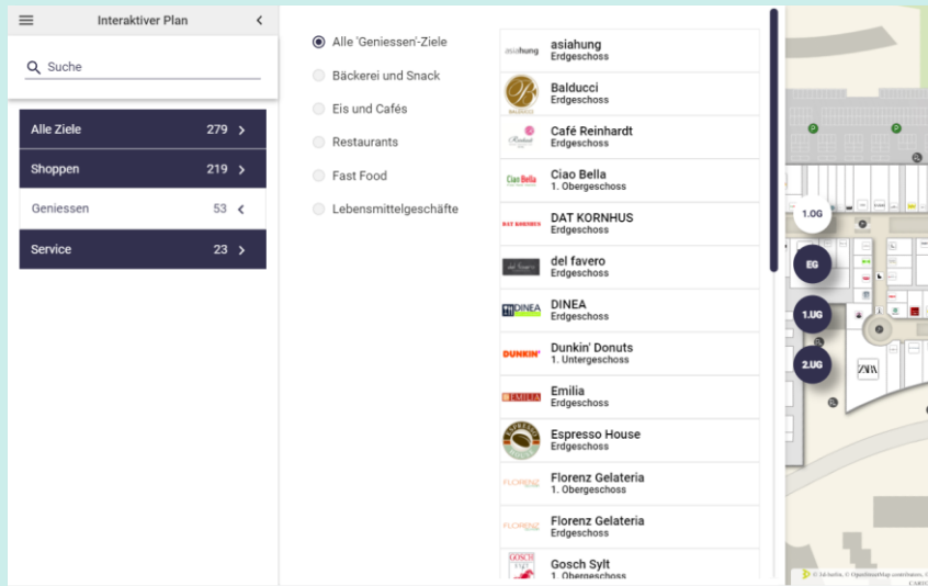
Kategoriesuche
